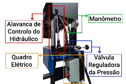
Distribuidor Manual
